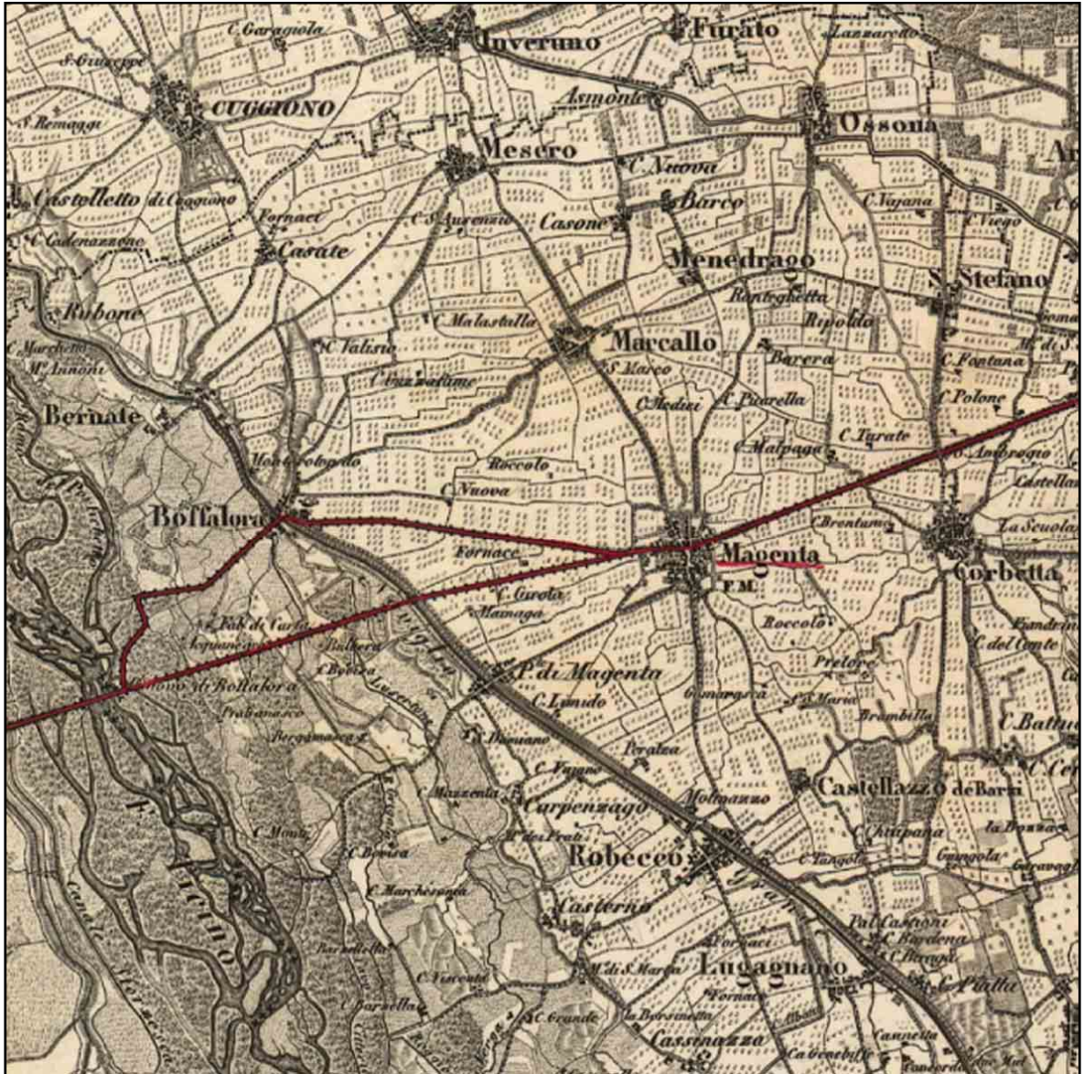
Fig. 2. IGM austriaco, carta topografica del Regno Lombardo Veneto". Vienna, incisione 1833-1856, scala originaria 1:86.400. Fonte: archivio e biblioteca dell'IGM, Firenze.
