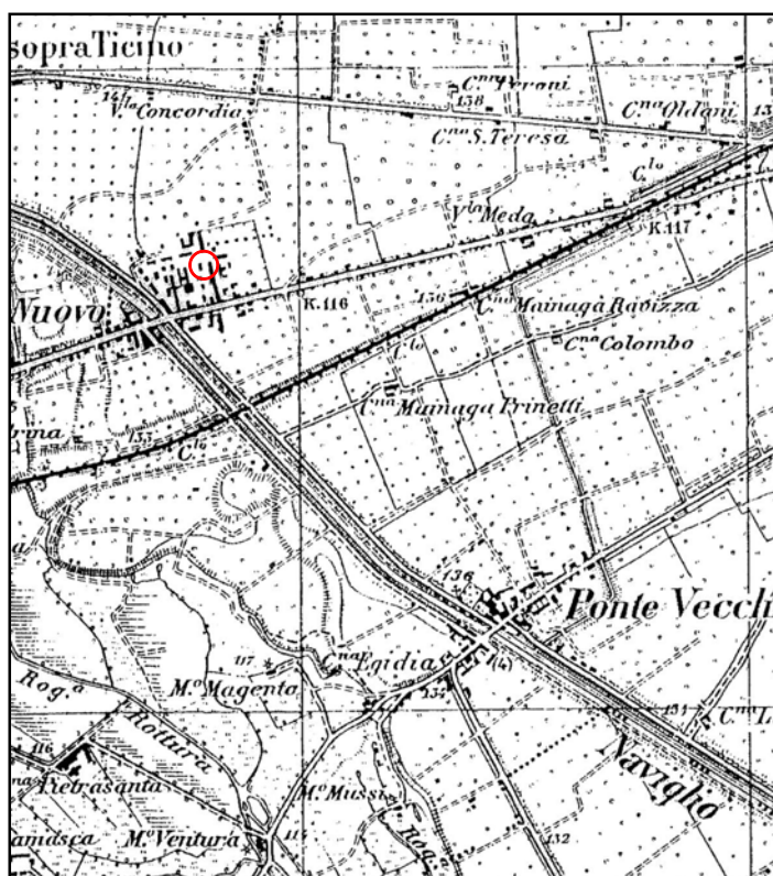
Fig. 38. IGM, tavoletta Magenta", 1933. Scala 1:20.000 circa. Estratto di Ponte Nuovo e Ponte Vecchio.
