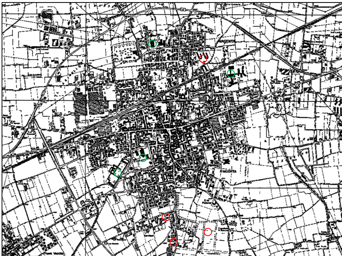
Fig. 46. Carta Tecnica Regionale (CTR), 1982.
